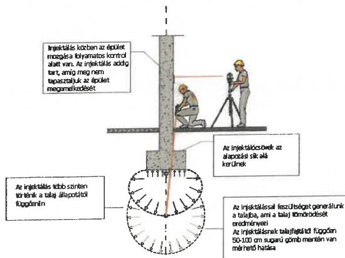
3. ábra Az injektálás mintakeresztmetszete
